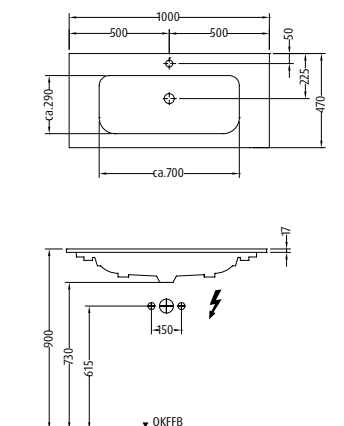
SL241/SL251
