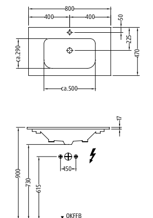
SL240/SL250
