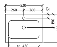
SY220/SY230
