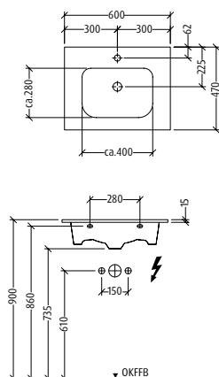
SL244/SL254
