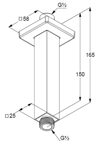
Maßzeichnung/ Dimensional drawing
