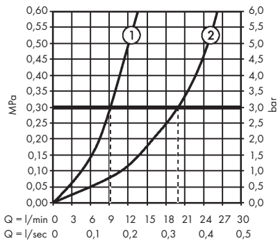
AXOR Edge 46430XXX/46431XXX
