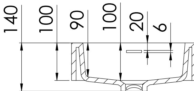
SCHNITT A-A
