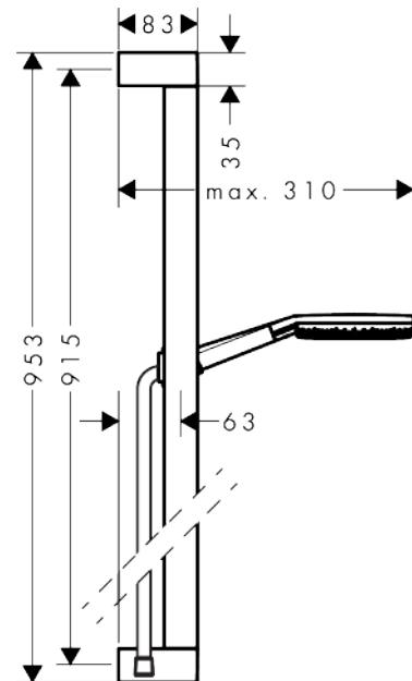
Maßzeichnung
