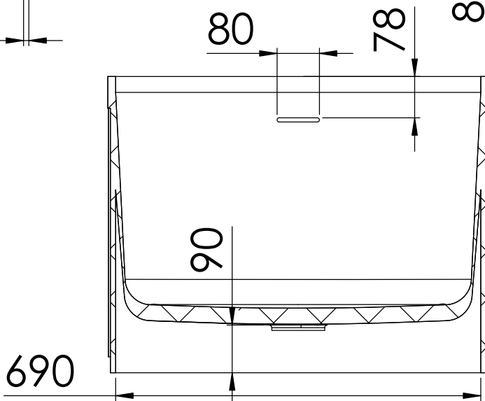
Schnitt B-B
