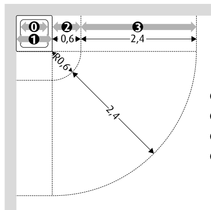
Bereichseinteilung bei Räumen mit Duschwanne
